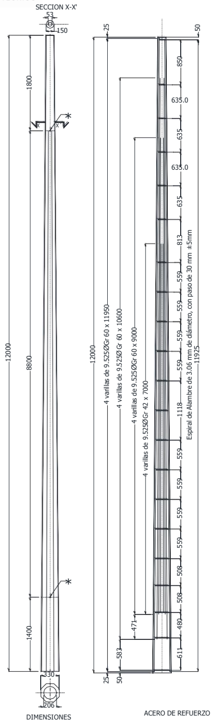
FIGURA 5- Poste PCRGR60-12-750
